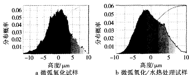
图4 钛合金微弧氧化层微孔深度分布特征
