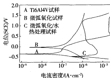
图6 钛合金及经过表面处理钛合金的动电位极化曲线
