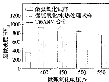
图5 钛合金微弧氧化层水热处理前后的显微硬度
