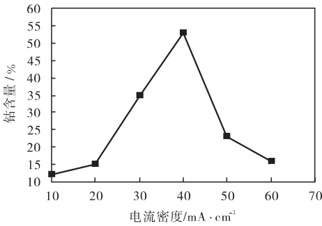
图3 电流密度对镀层中钴含量的影响
