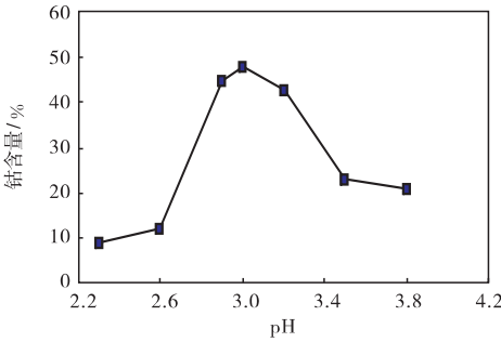
图4 pH对镀层中钴含量的影响
